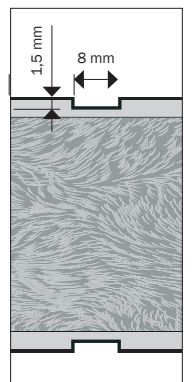
Detail drážky dverí Siluet
