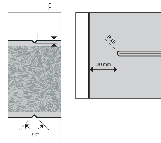
Detail drážky „V“ dverí Element
