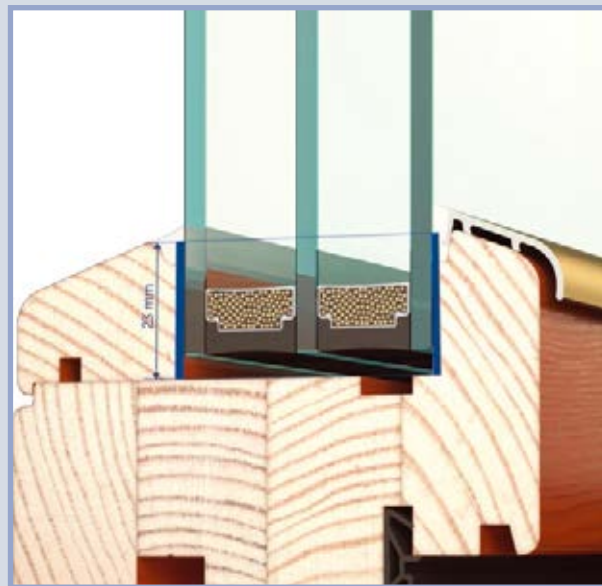
tiefer Verglasungsfalz
