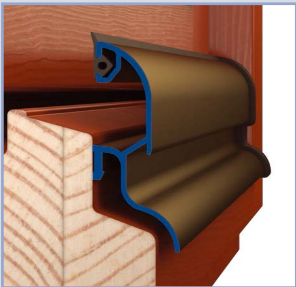
Rahmenregenschiene
